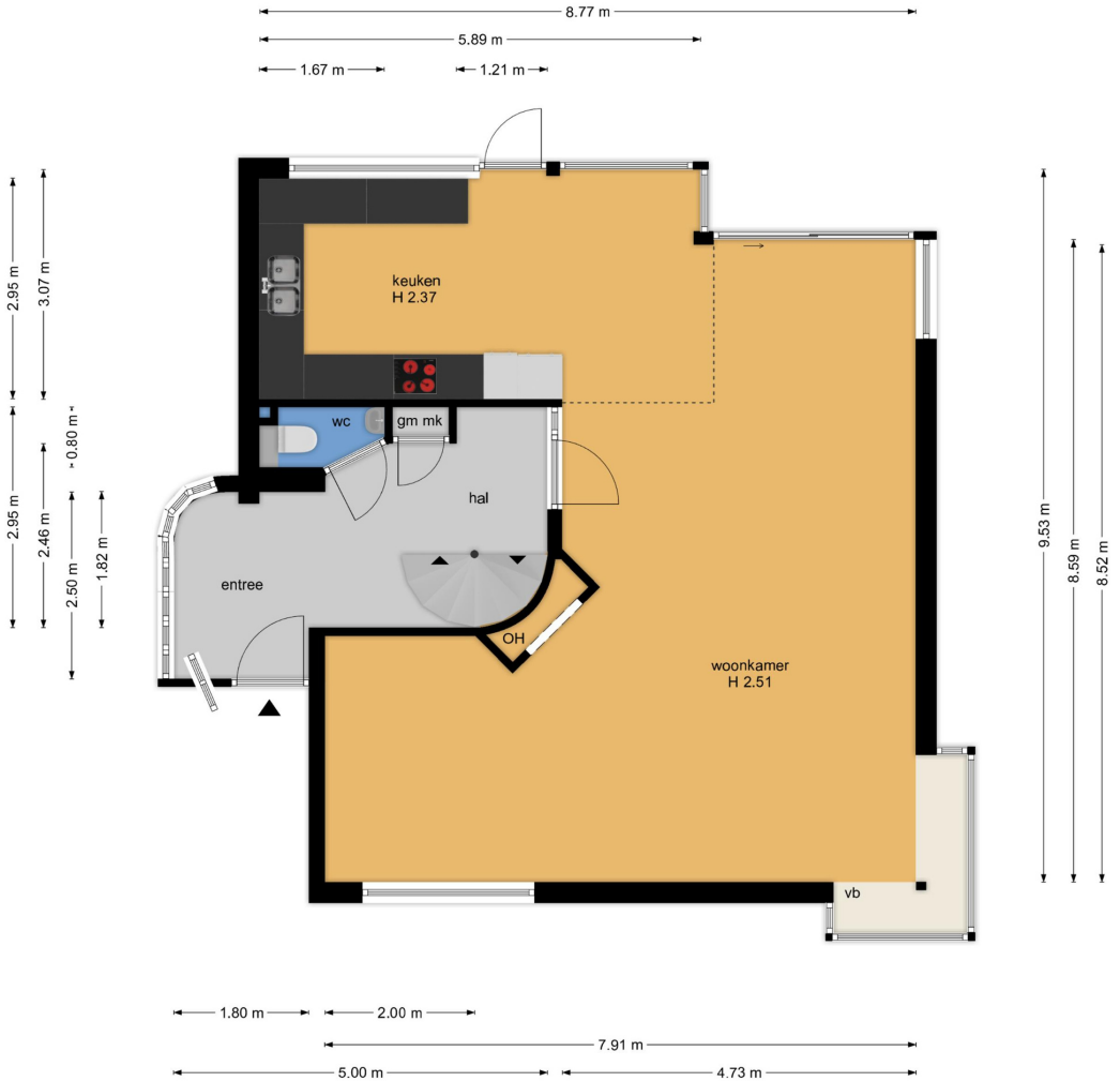
begane grond
